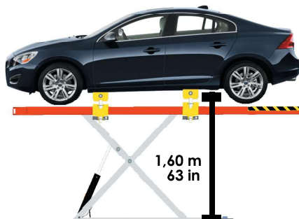
Levage par les bas de caisse Lifting from rocker panels
